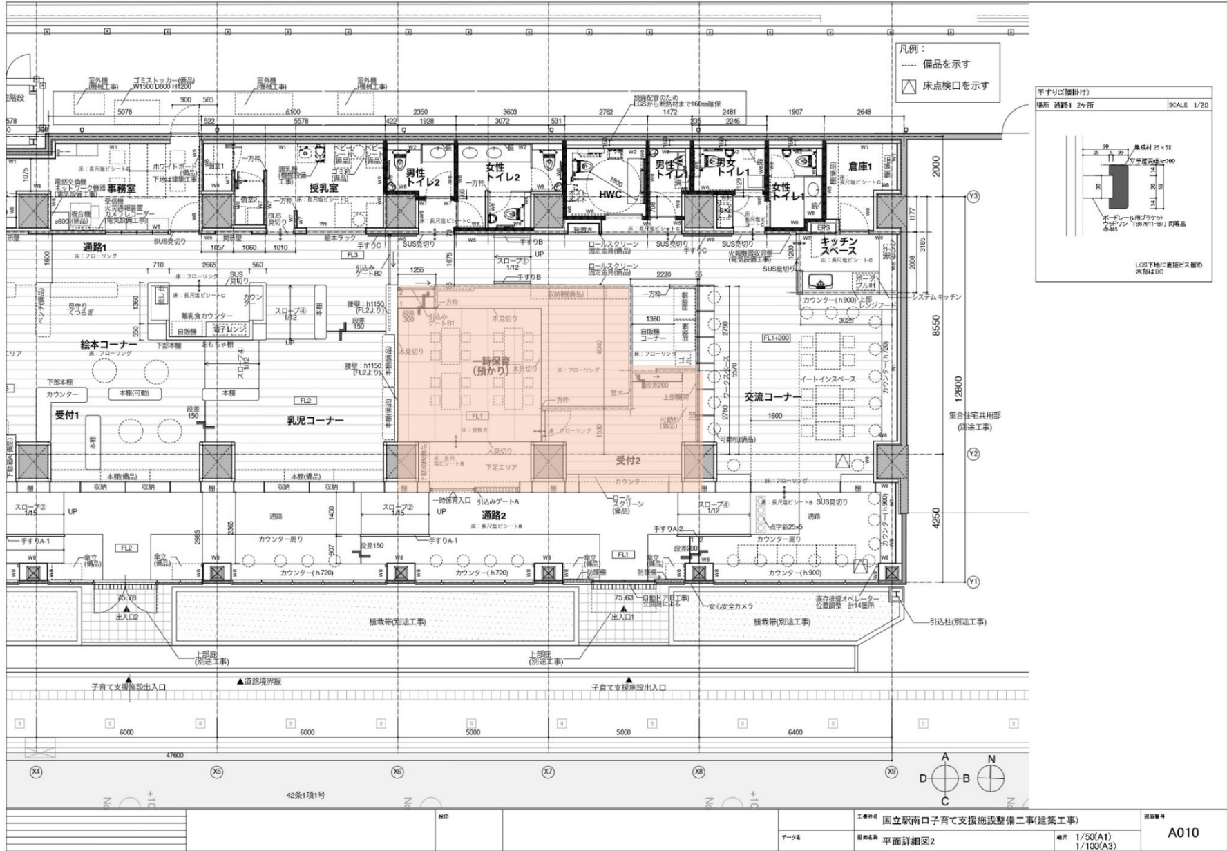
平面図 (拡大)
