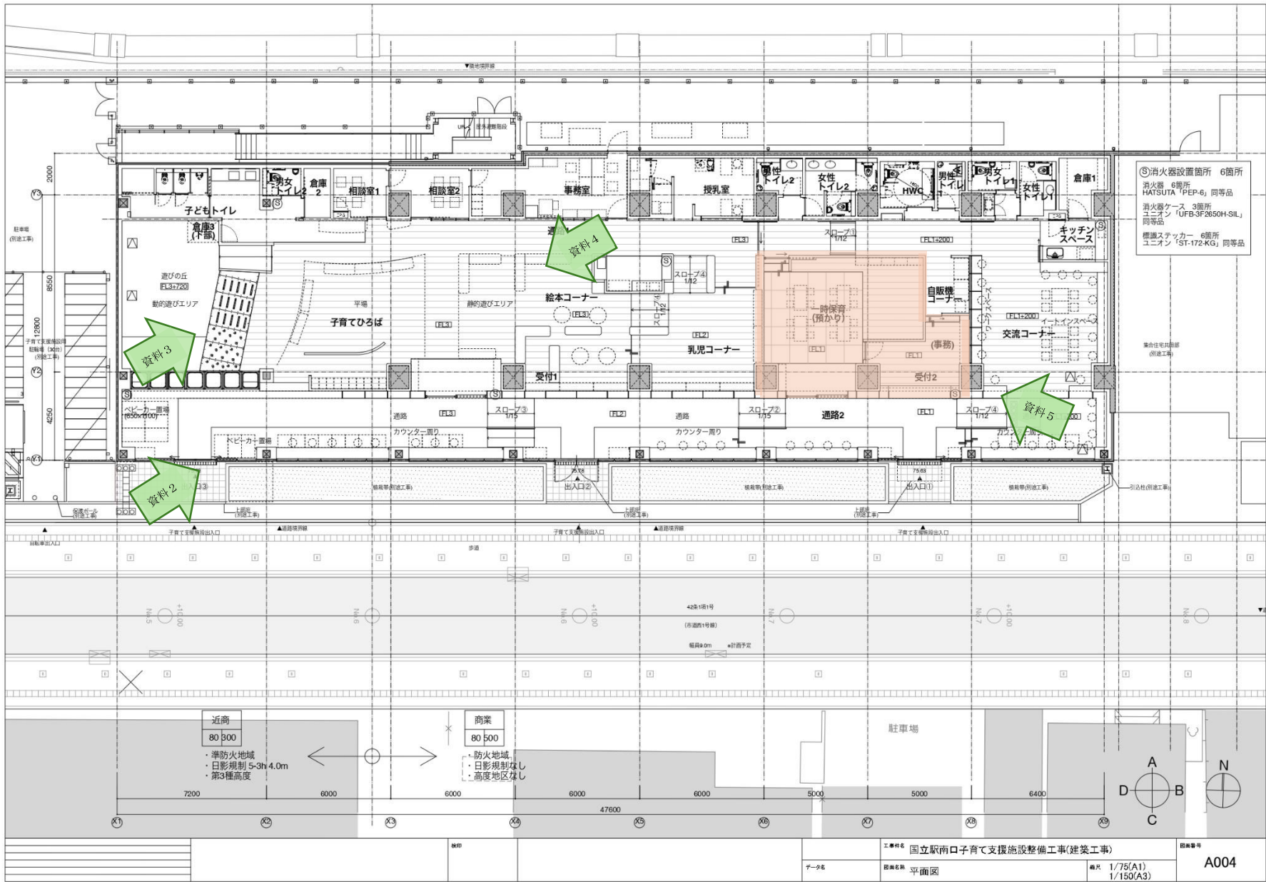
平面図
